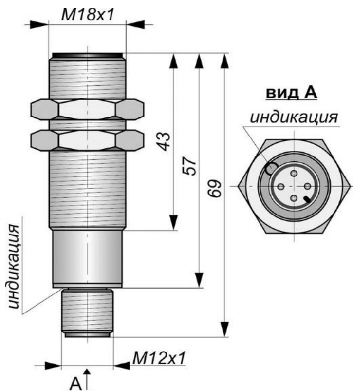
Габаритный чертеж
