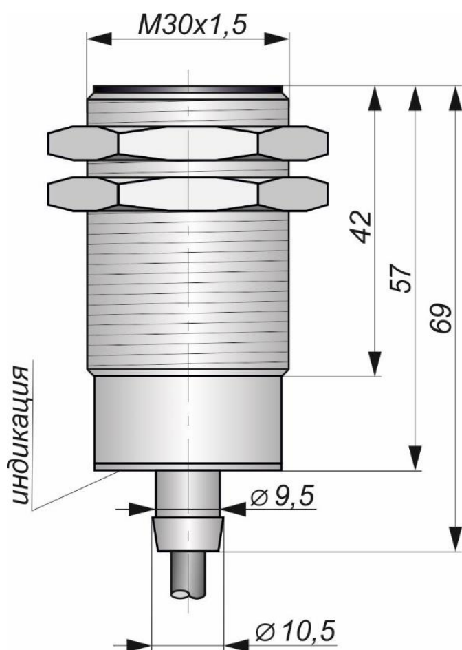
Габаритный чертеж
