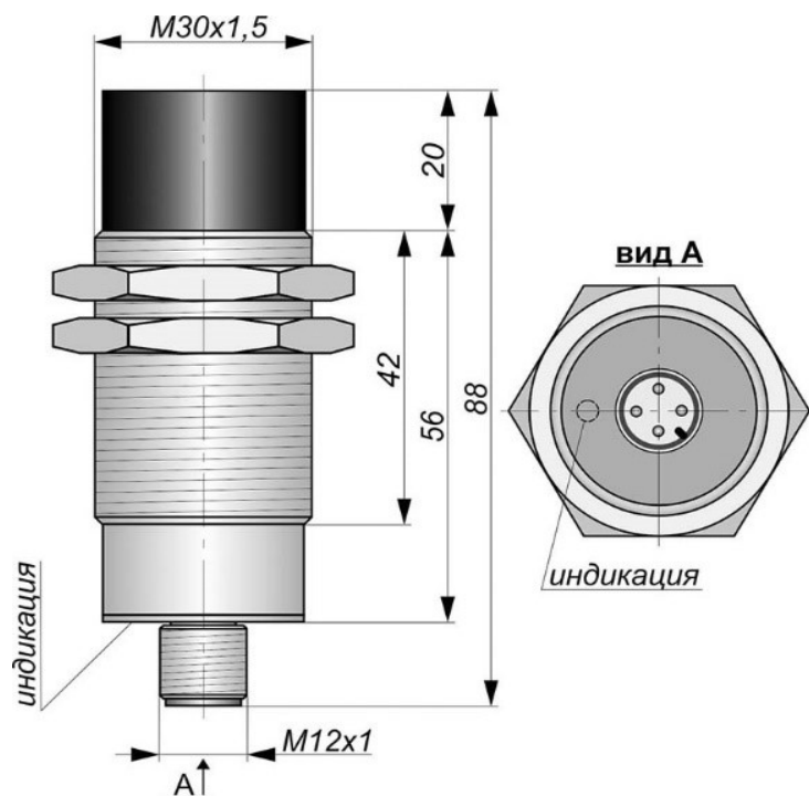
Габаритный чертеж
