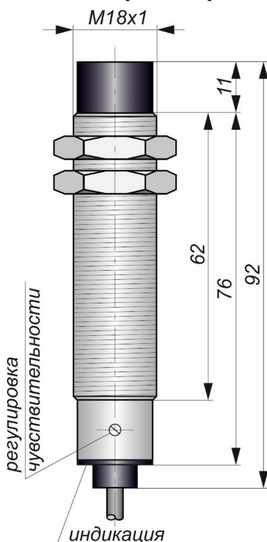
Габаритный чертеж
