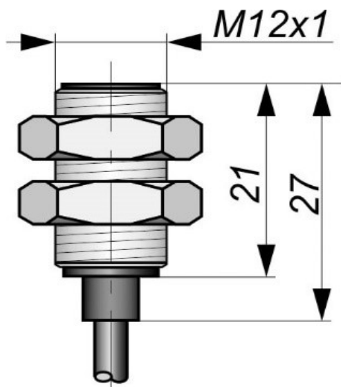
Габаритный чертеж
