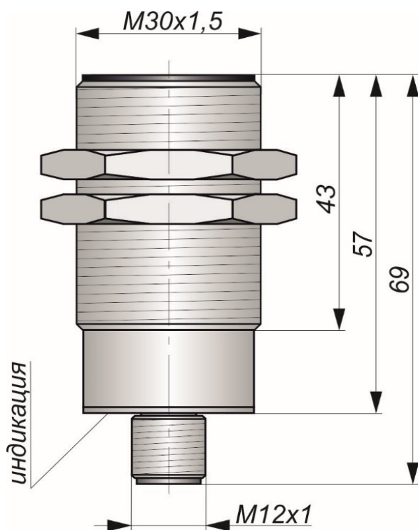
Габаритный чертеж
