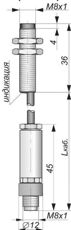
Габаритный чертеж
