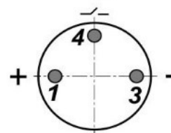
Цоколевка разъема
