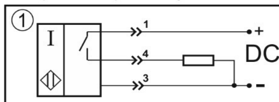
Схема соединения Нормально-разомкнутый контакт
