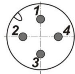
Цоколевка разъема
