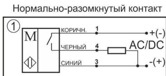
Схема соединения
