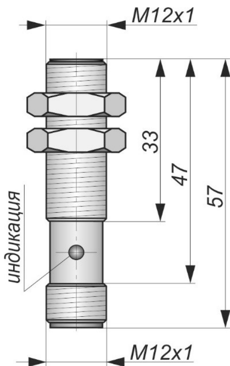
Габаритный чертеж
