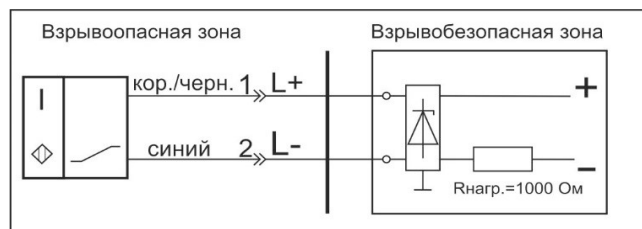
Цоколевка разъема
