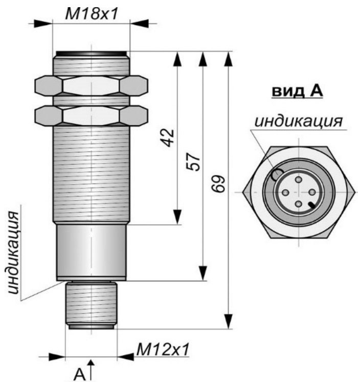
Габаритный чертеж
