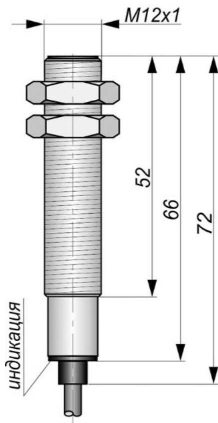
Габаритный чертеж
