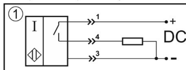
Нормально-разомкнутый контакт
