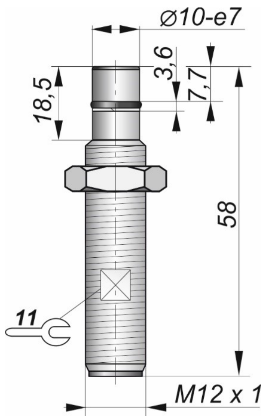
Габаритный чертеж
