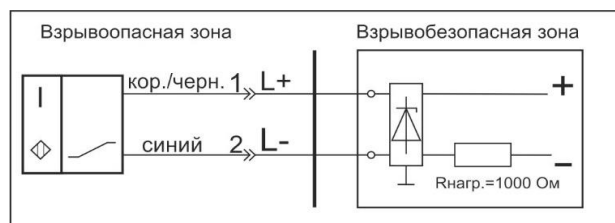
Схема соединения
