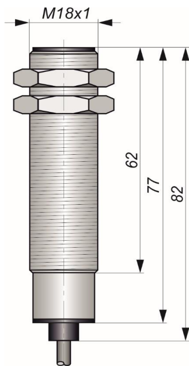
Габаритный чертеж
