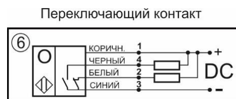
Схема соединения
