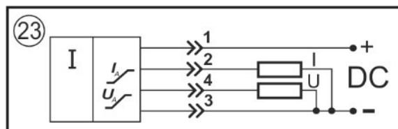
Схема соединения
