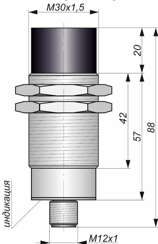
Габаритный чертеж
