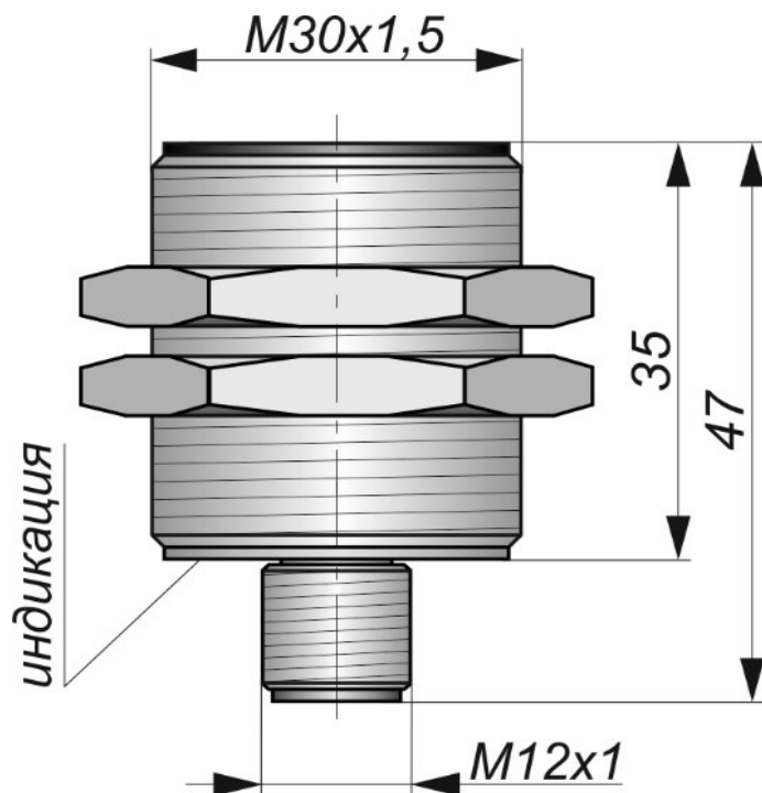
Габаритный чертеж
