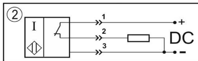
Цоколевка разъема
