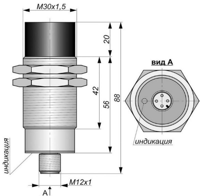
Габаритный чертеж
