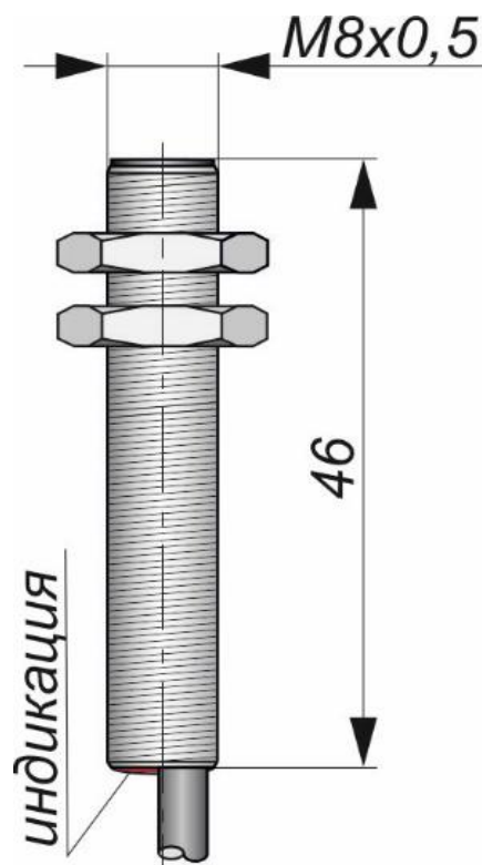
Габаритный чертеж
