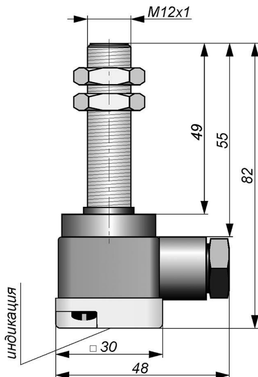
Габаритный чертеж
