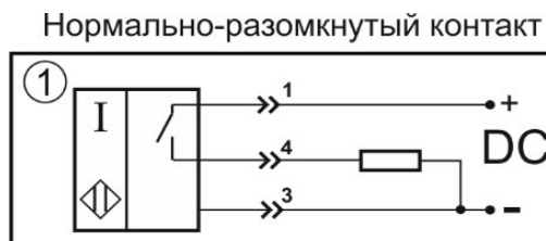
Цоколевка разъема
