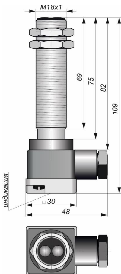
Габаритный чертеж
