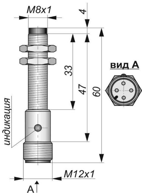
Габаритный чертеж
