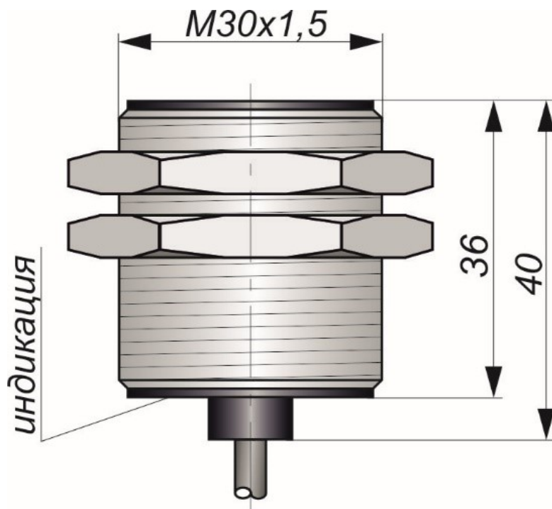
Габаритный чертеж
