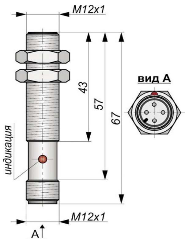
Габаритный чертеж
