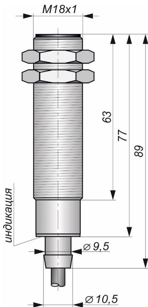
Габаритный чертеж
