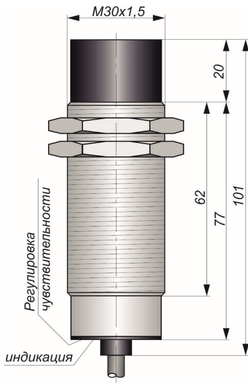
Габаритный чертеж
