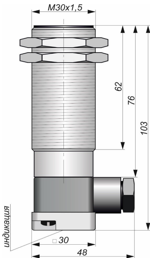
Габаритный чертеж
