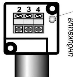
Цоколевка клеммной колодки
