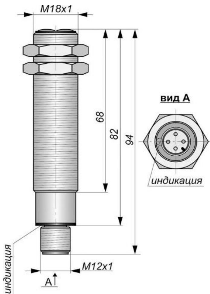
Габаритный чертеж
