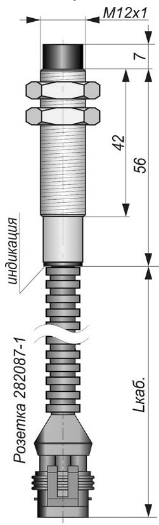
Габаритный чертеж
