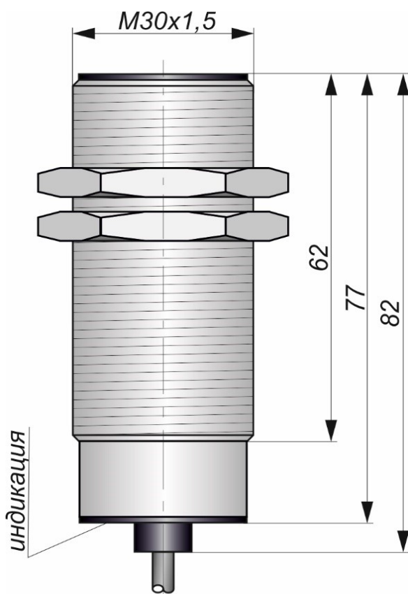
Габаритный чертеж
