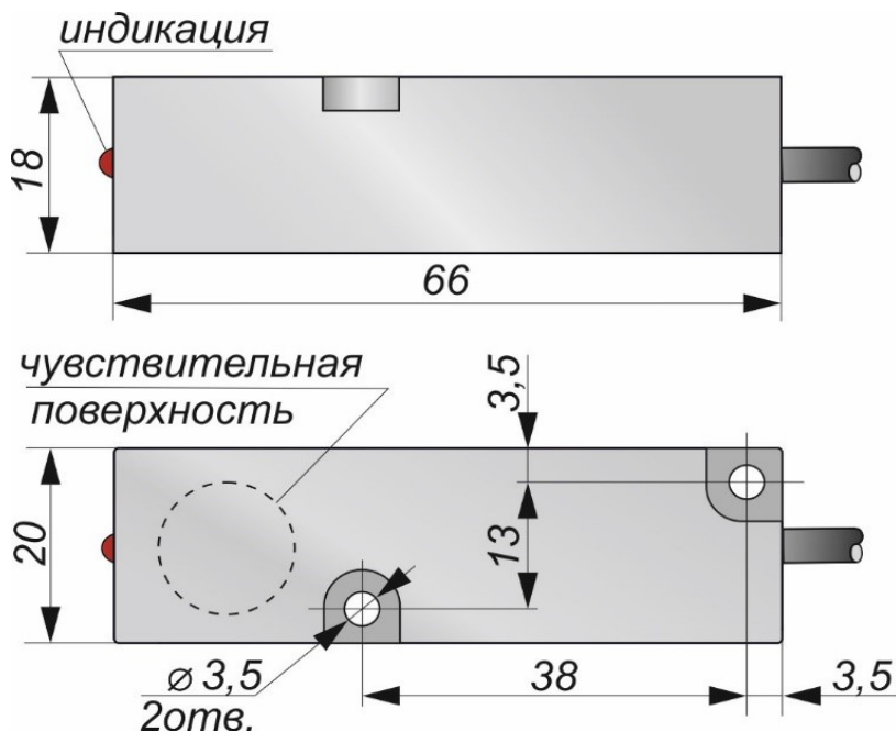
Габаритный чертеж
