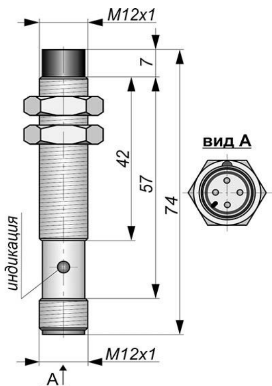
Габаритный чертеж
