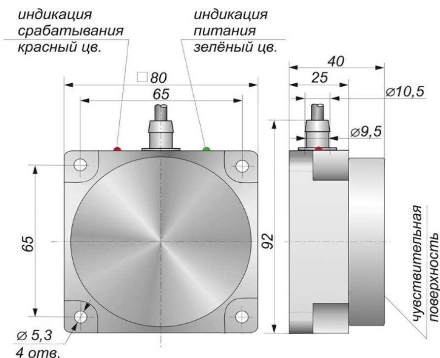
Габаритный чертеж
