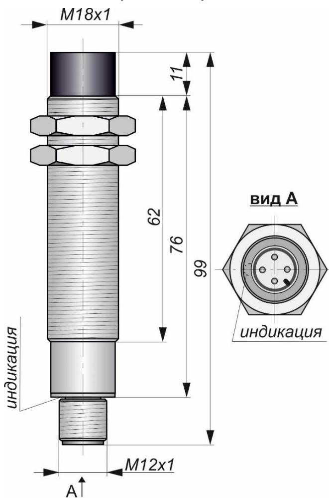
Габаритный чертеж
