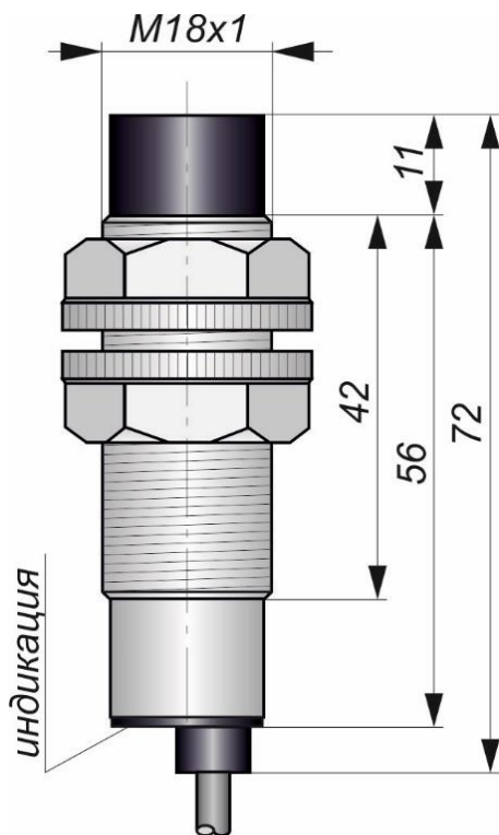
Габаритный чертеж
