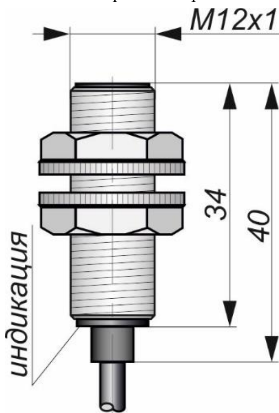
Габаритный чертеж
