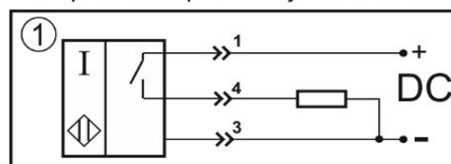
Цоколевка разъема
