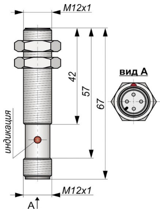
Габаритный чертеж
