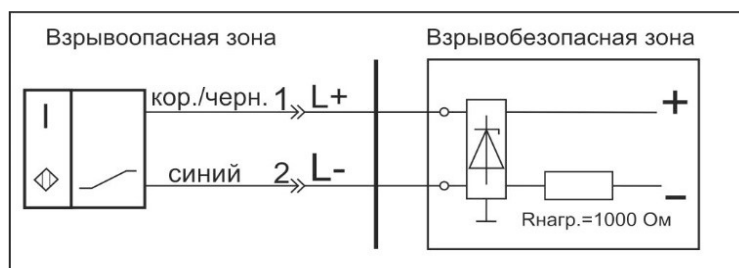
Схема соединения
