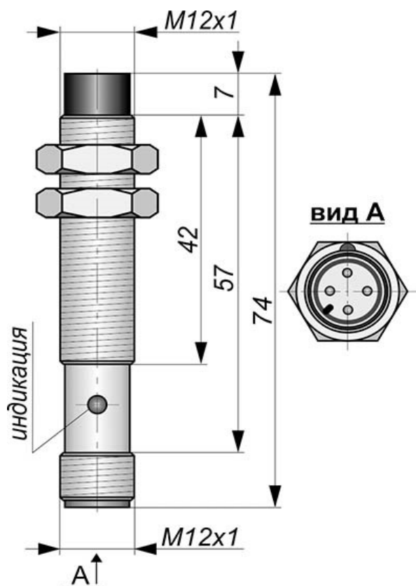
Габаритный чертеж
