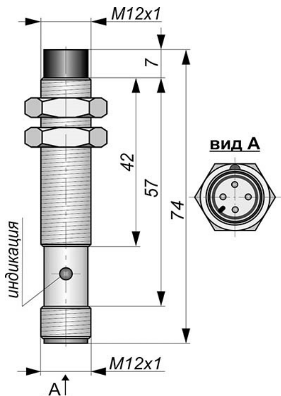
Габаритный чертеж
