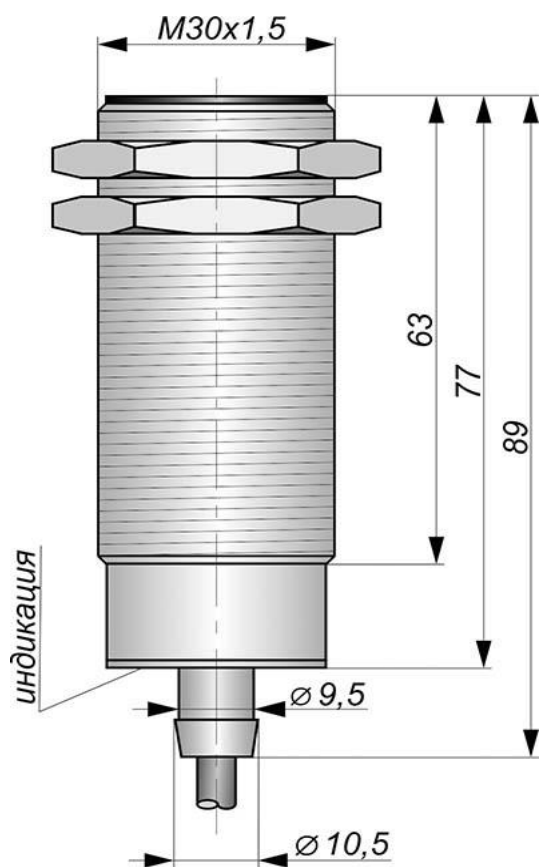
Габаритный чертеж
