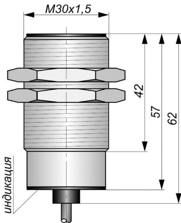
Габаритный чертеж
