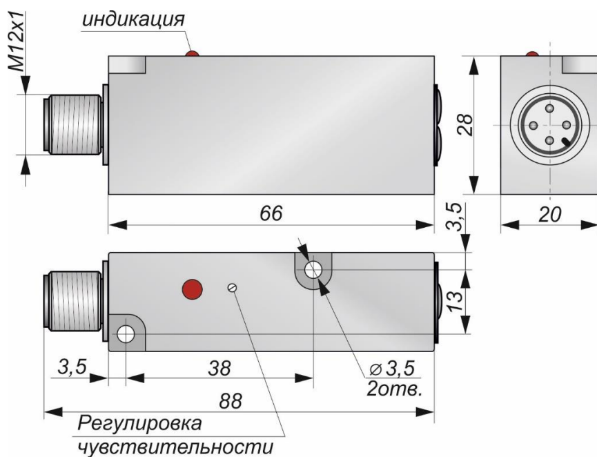
Габаритный чертеж
