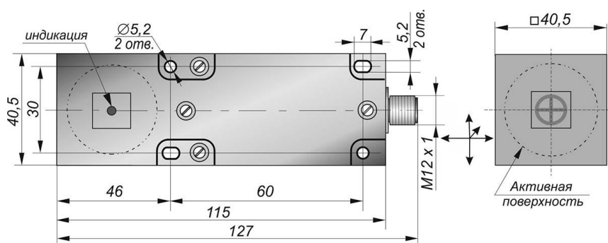
Габаритный чертеж
