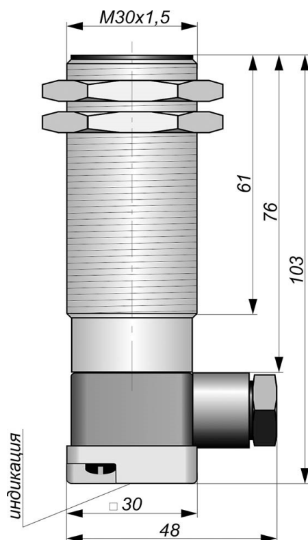
Габаритный чертеж
