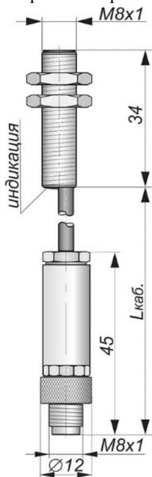
Габаритный чертеж
