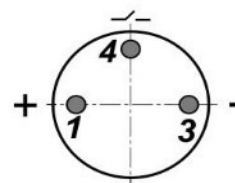
Цоколевка разъема
