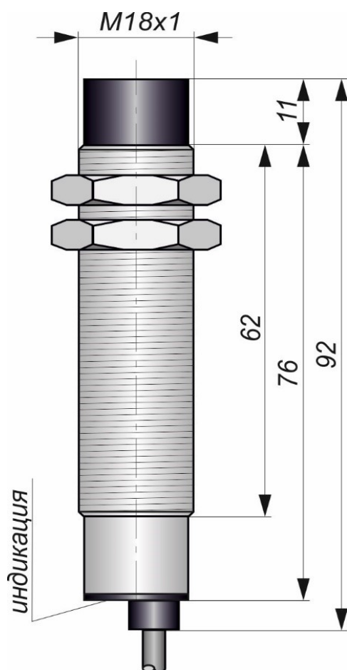
Габаритный чертеж
