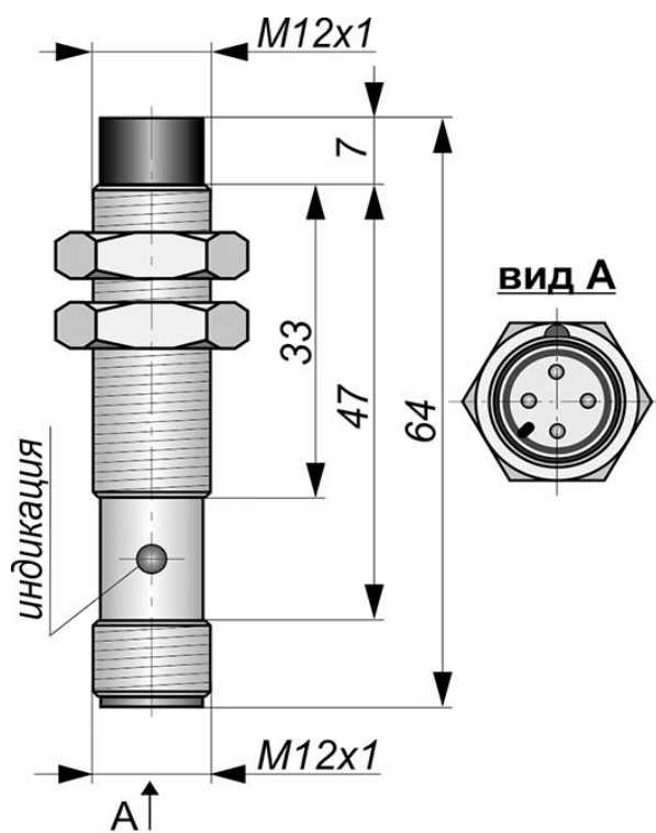
Габаритный чертеж
